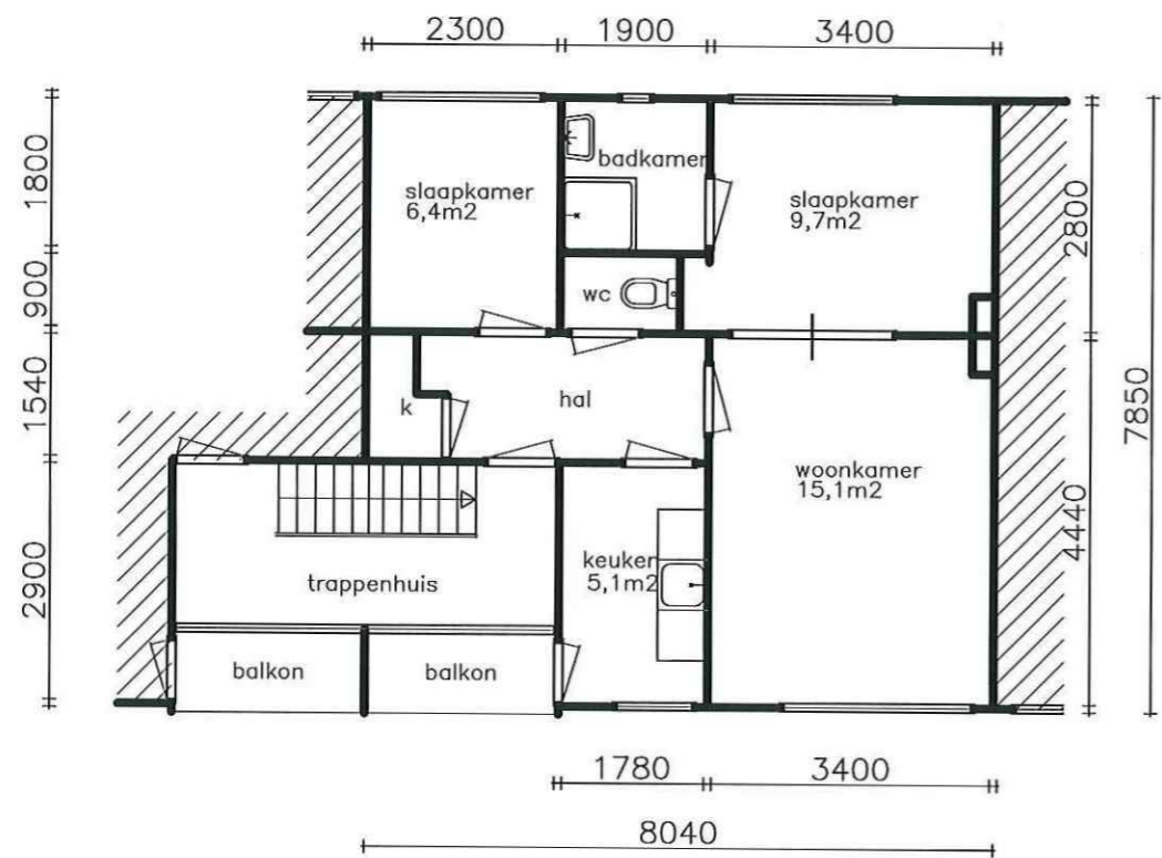
1E VERDIEPING
