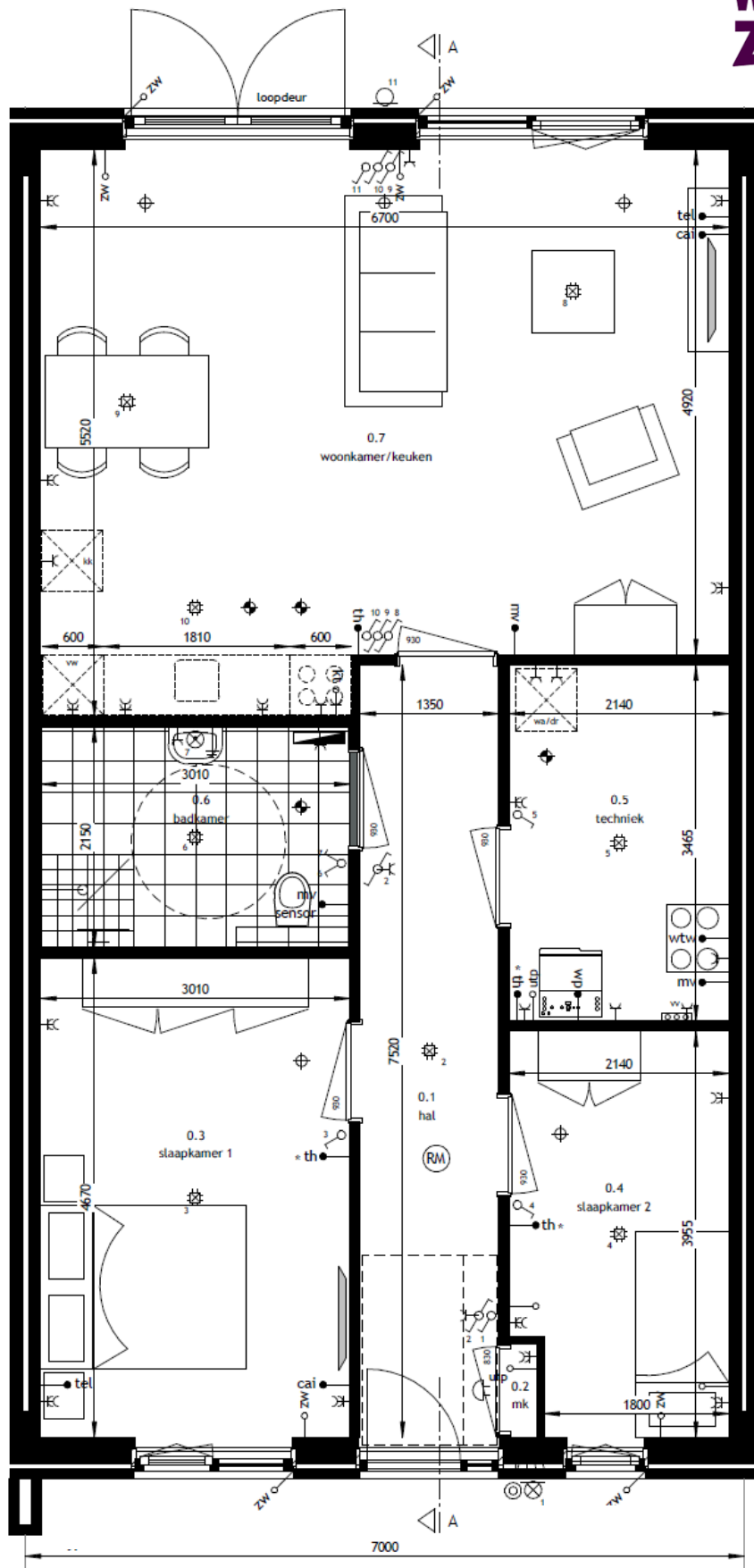
Begane Grond Nultredenwoning
